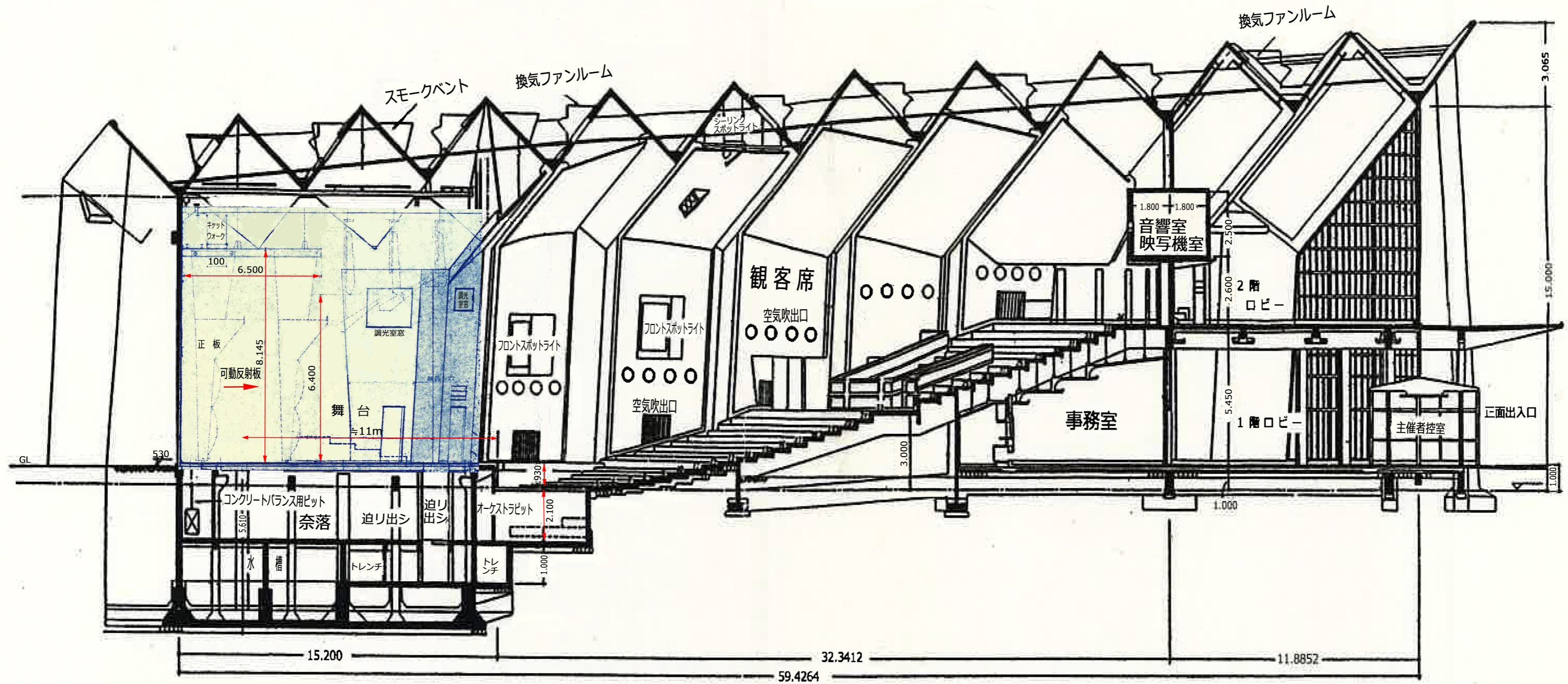
縦断面図 section 1/300 ※音響反射板改修1988年
